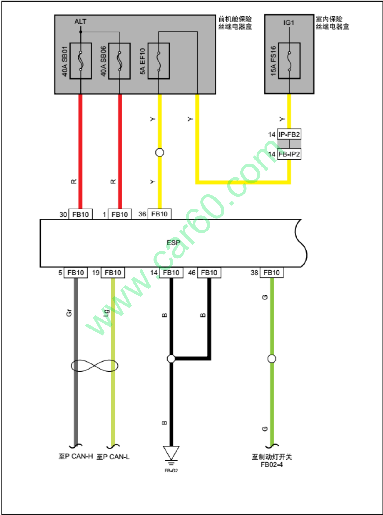
ABS ESP电源、接地、数据线1
